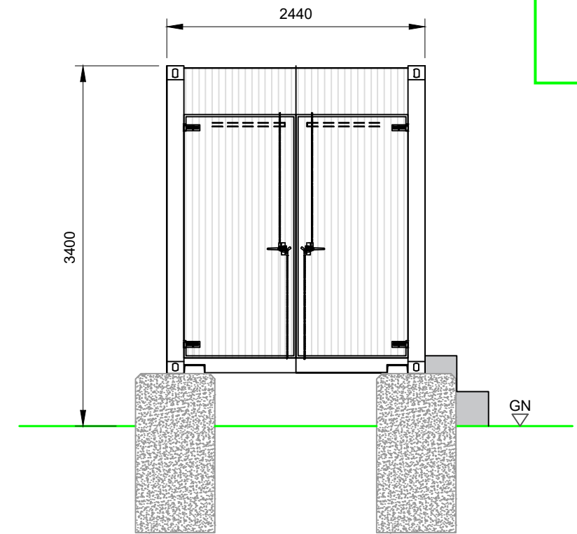
Zijaanzicht
