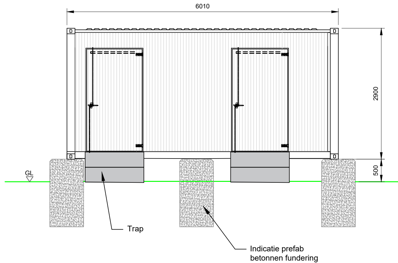
Voorraanzicht
