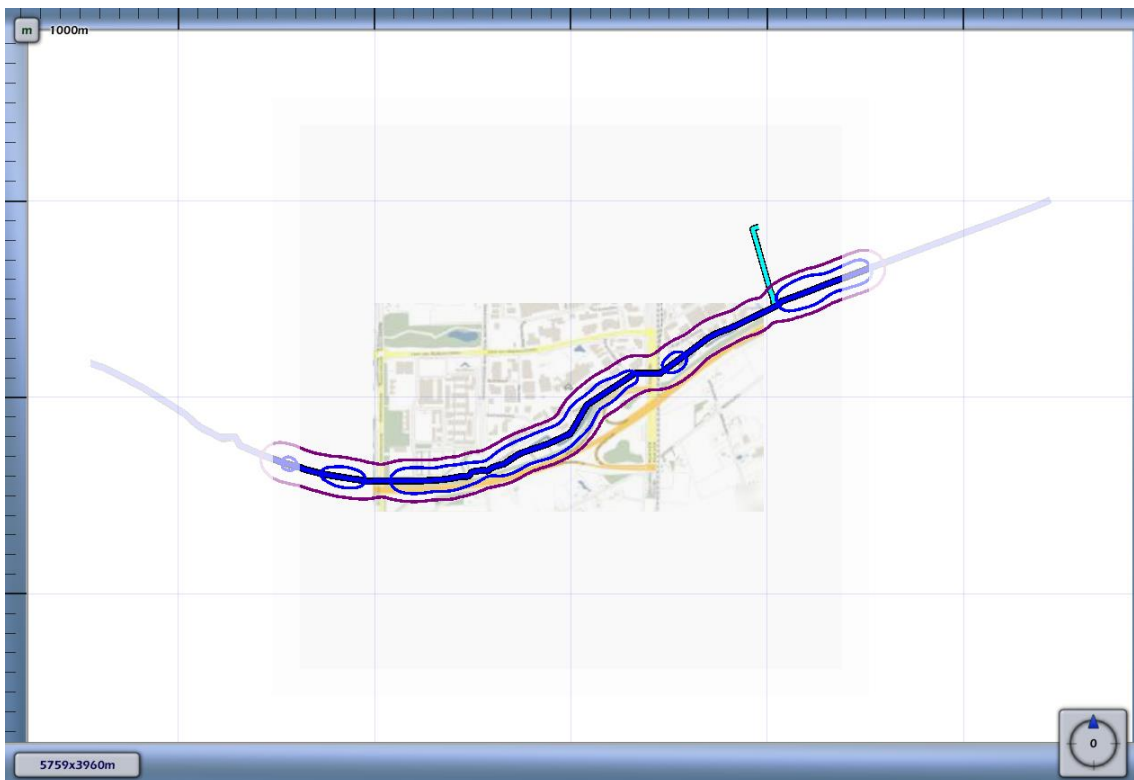
3.1 Figuur 3.1 Plaatsgebonden risico voor leiding-N-552-70-deel-1 van N.V. Nederlandse Gasunie
