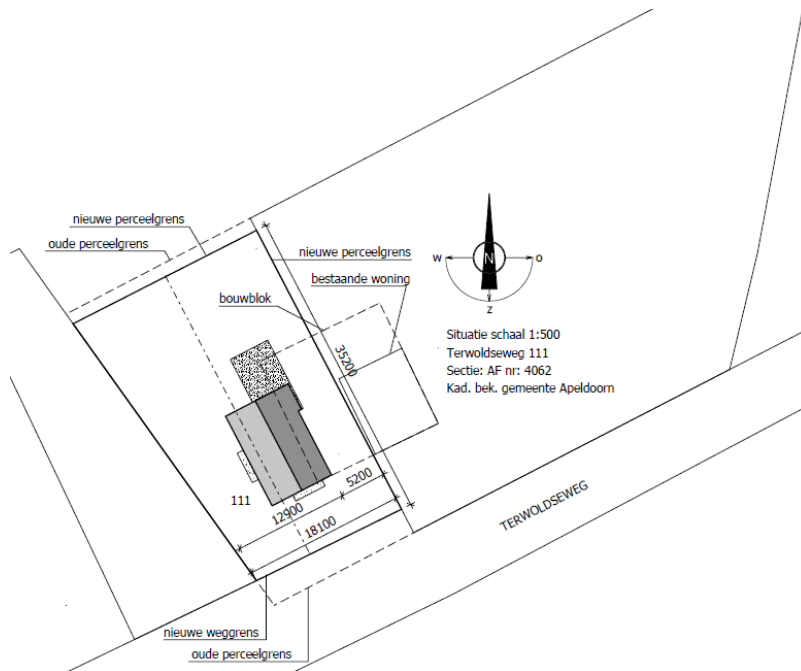
Figuur 4: Situatietekening nieuwe woning
