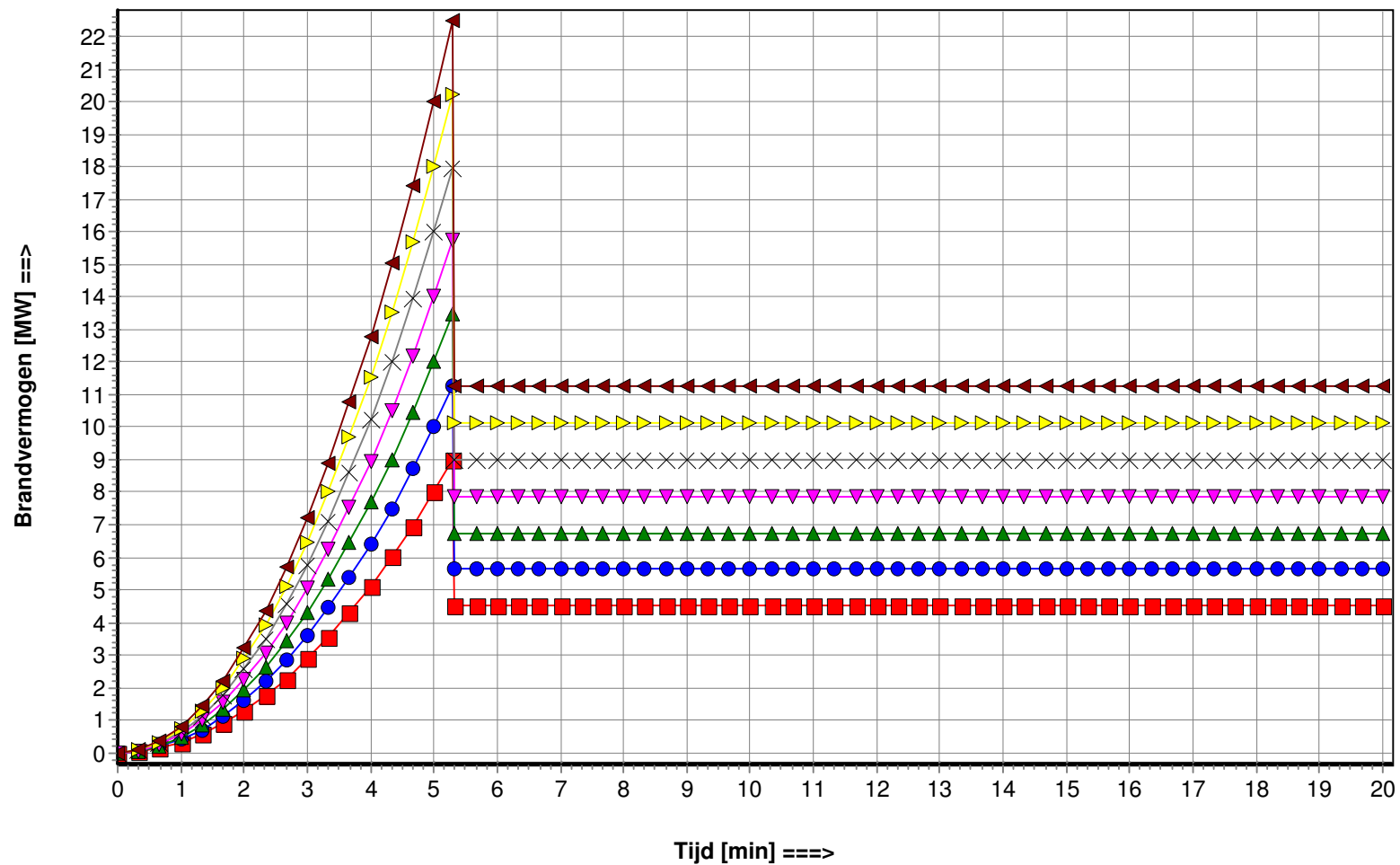
Brandvermogen als functie van de tijd
