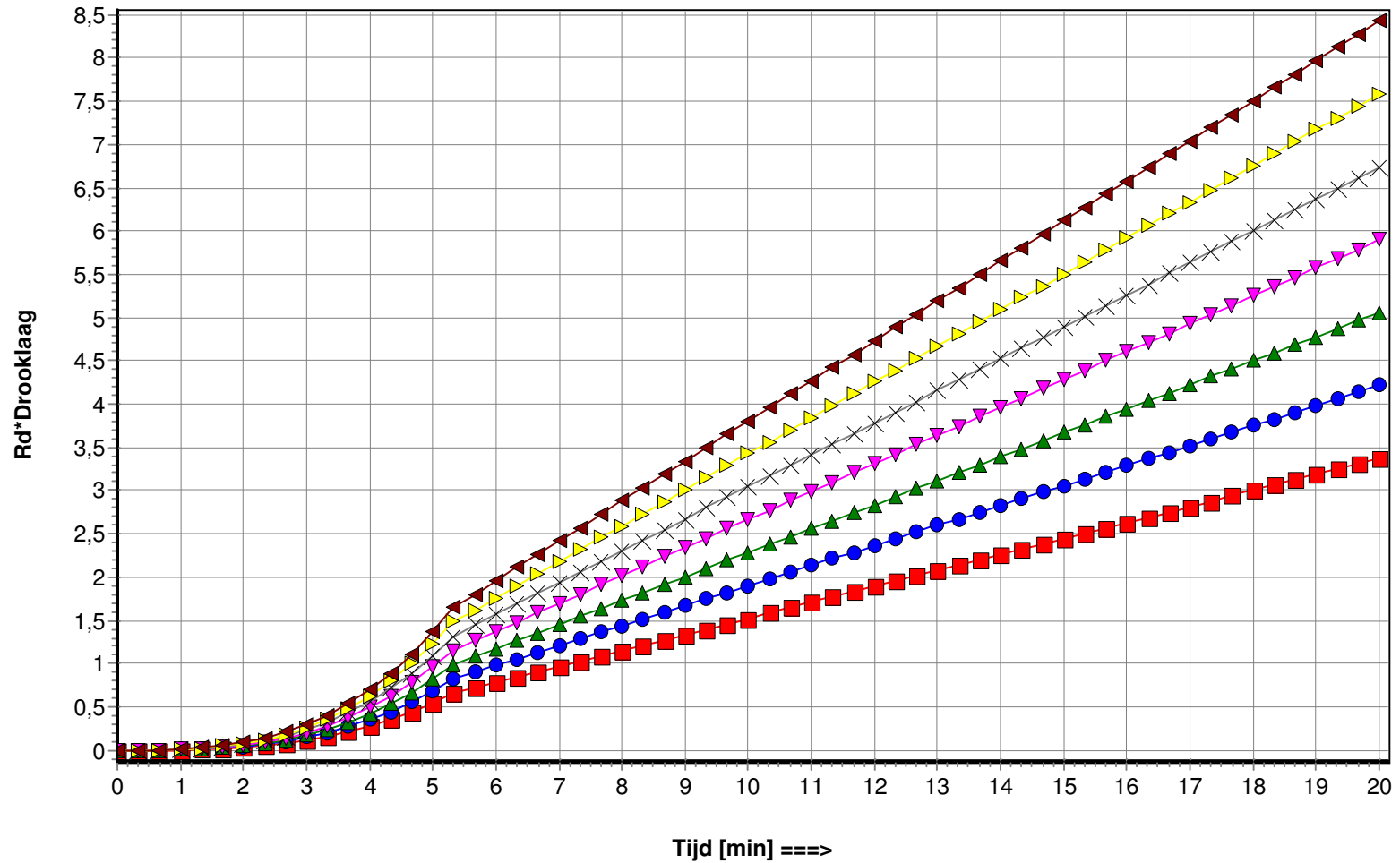
Rd*Drooklaag als functie van de tijd
