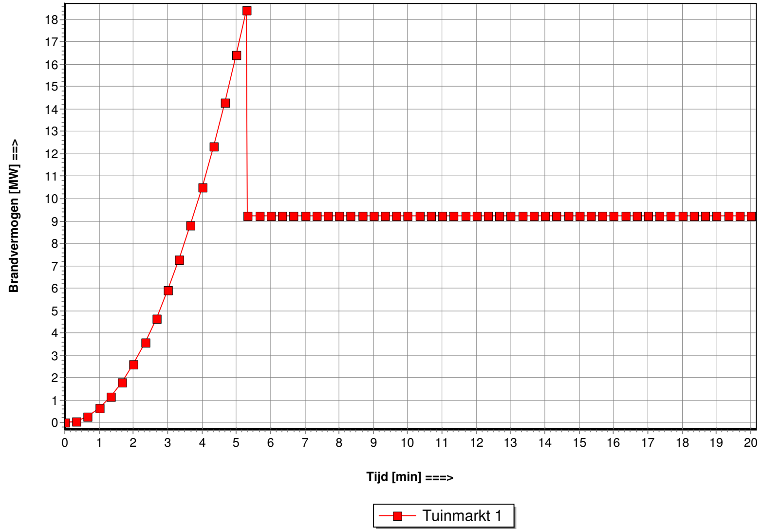
Brandvermogen als functie van de tijd
