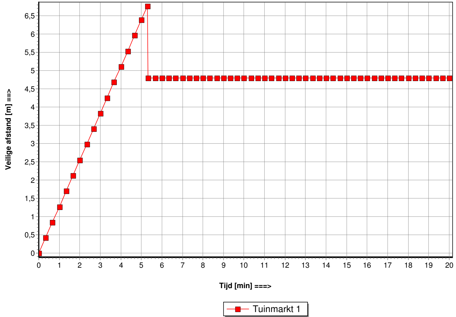
Veilige afstand als functie van de tijd
