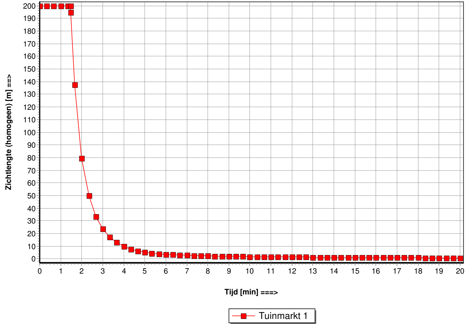
Zichtlengte (homogeen) als functie van de tijd
