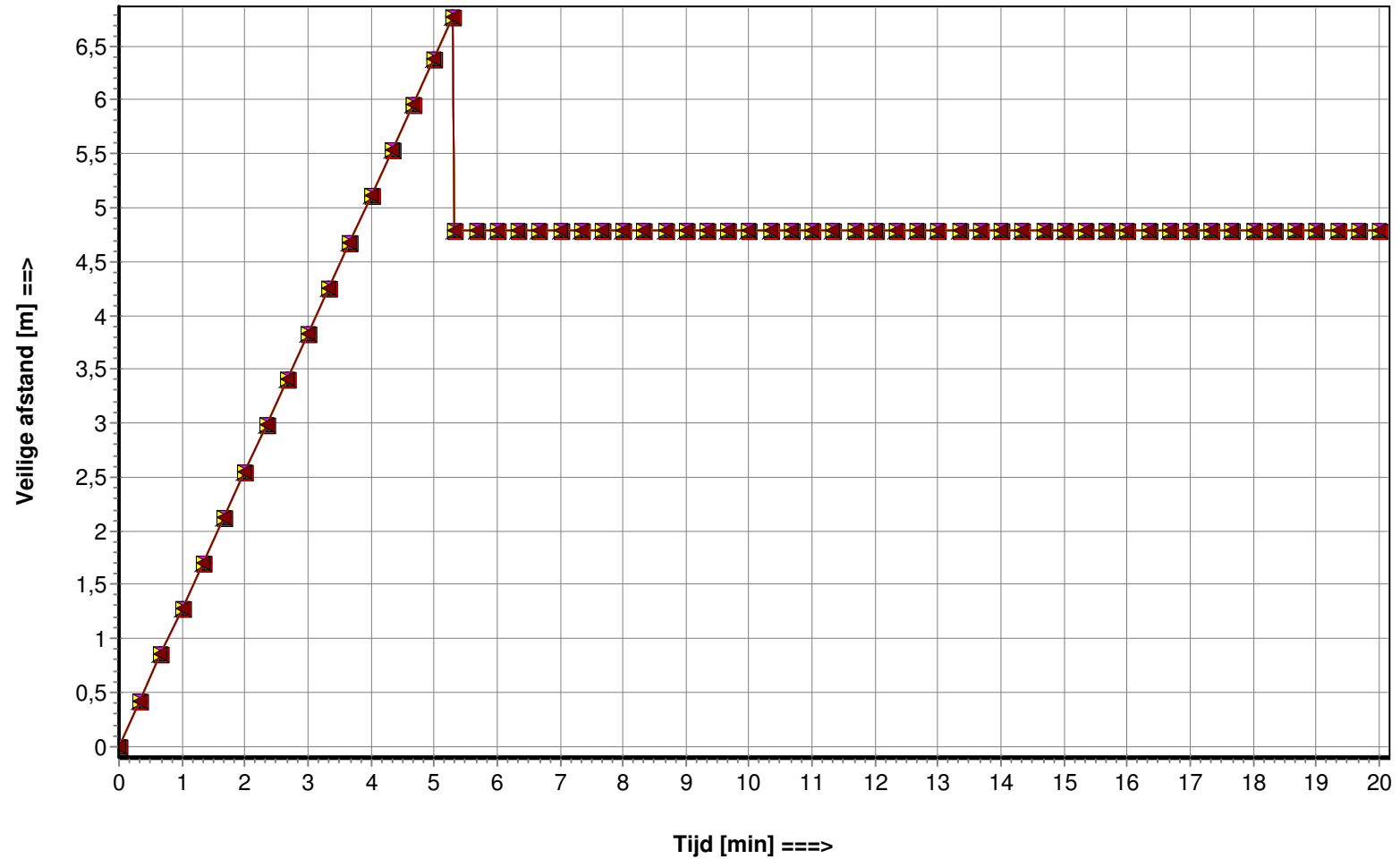
Veilige afstand als functie van de tijd
