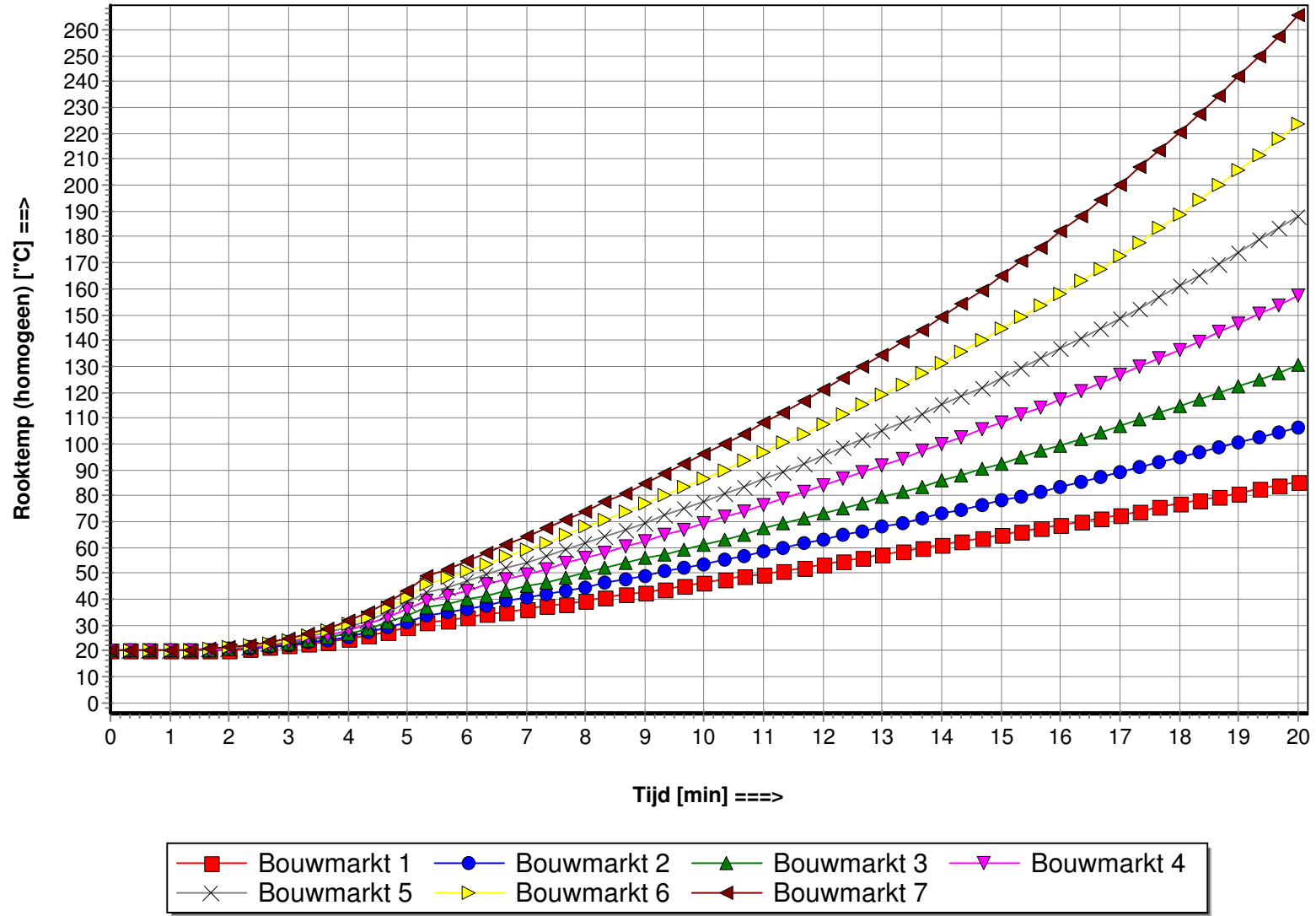
Rooktemp (homogeen) als functie van de tijd
