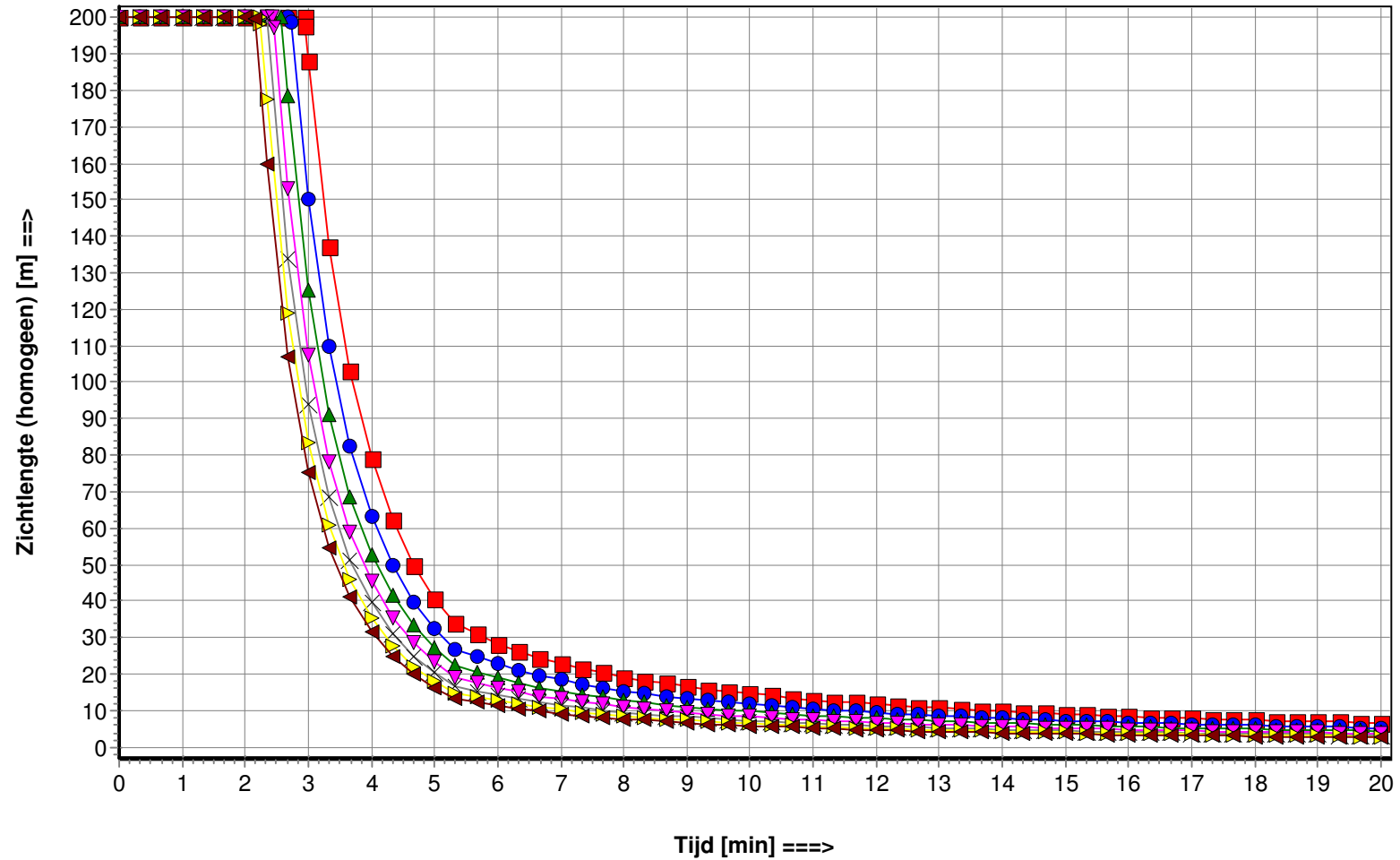
Zichtlengte (homogeen) als functie van de tijd
