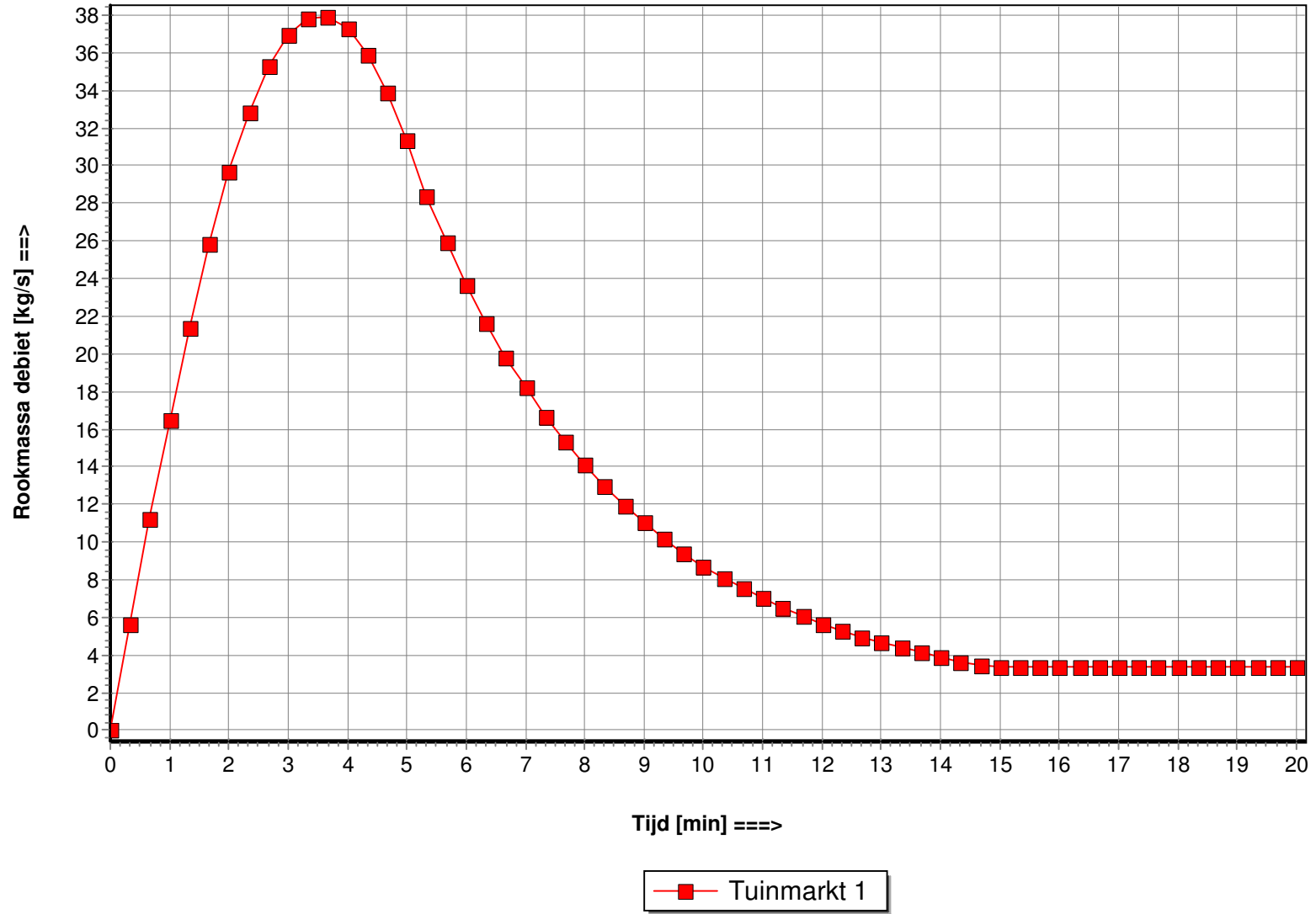
Rookmassa debiet als functie van de tijd
